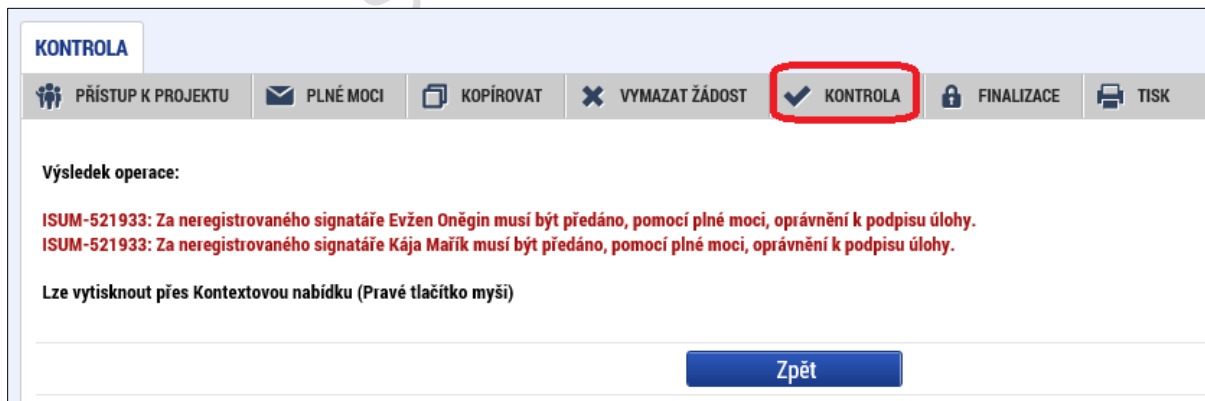
Obrázek 66: Kontrolní hláška
